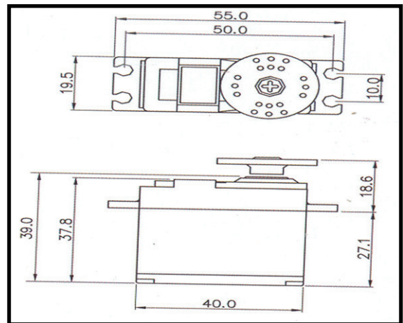
Servos
